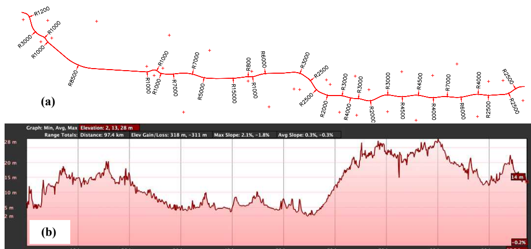
Gambar 2. (a) Kelengkungan Rute Non-Tol dan (b) Kelandaian Rute Jalan Tol
