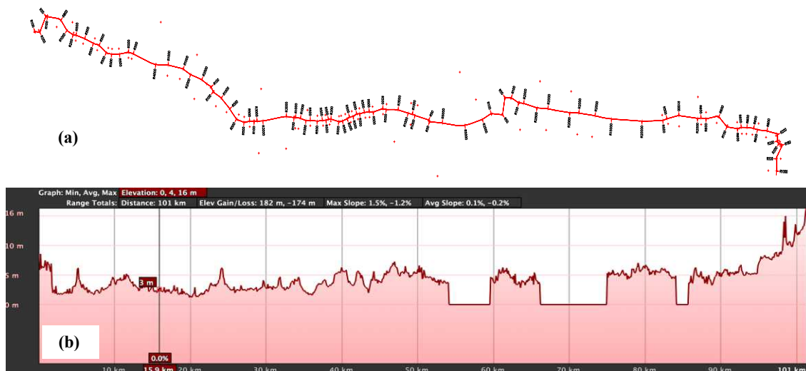
Gambar 3. (a) Kelengkungan Rute Non-Tol dan (b) Kelandaian Rute Non-Tol
