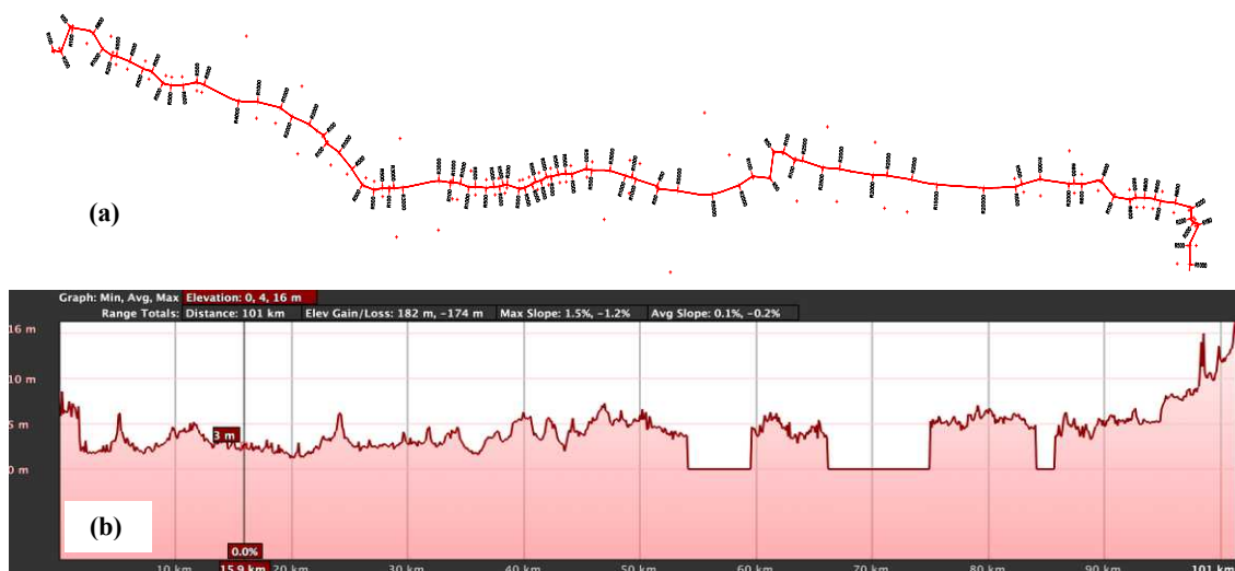
Gambar 6. (a) Kelengkungan Rute Non-Tol dan (b) Kelandaian Rute Non-Tol
